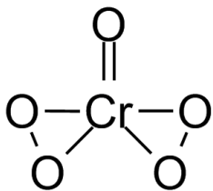
Chrom(VI)peroxid „Chromschmetterling“
