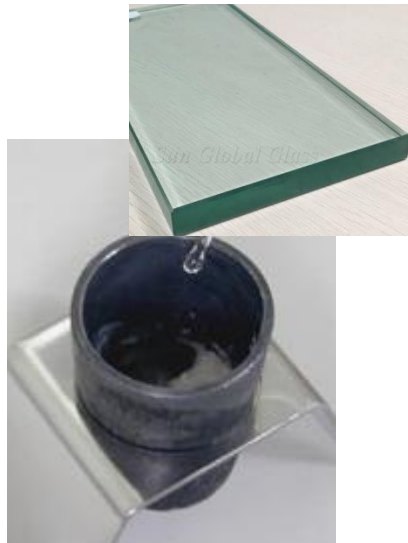
Ätzprobe
