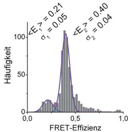
Abbildung 6.6.: Histogramm über die Mittelwerte zeitlich konstanter FRET-Effizienzen von 631 stabilen TBP-DNA-TOA-Komplexen einer Messreihe vor der Zugabe von NC2.
