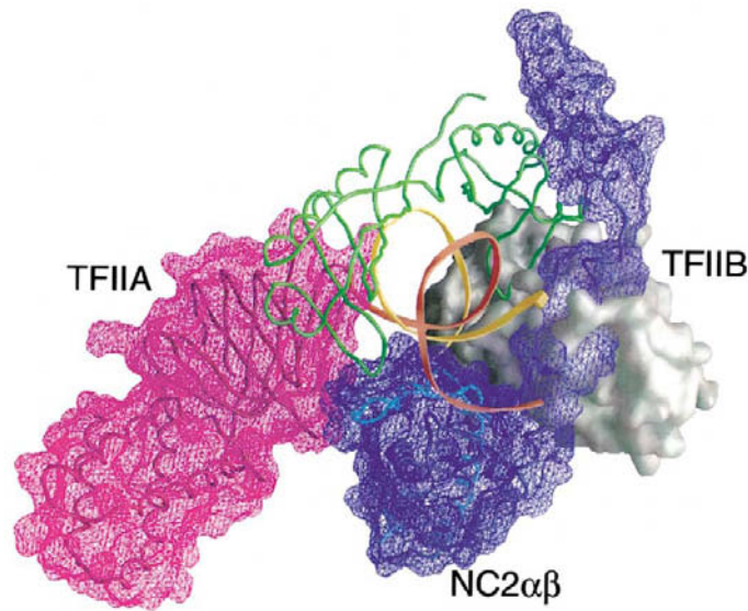
Abbildung 2.10.: Sterische Hinderung als möglicher Grund der Transkriptionshemmung durch NC2. Die Superposition der Kristallstrukturen der unterschiedlichen Komplexe von TBP(grün)-DNA(gelb und orange)-NC2(blau), TBP-DNA-TFIIA(rot) [38] und TBP-DNA-TFIIB(grau) [88] zeigt, dass NC2 die Bindung der Transkriptionsfaktoren IIA und IIB sterisch verhindert. Der C-Terminus der NC2 \alpha -Domäne ist in dieser NC2-Struktur nicht enthalten. (Abb. aus [3].)
