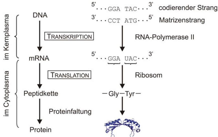
Abbildung 2.3.: Die Proteinbiosynthese von eukaryotischen Zellen. Im Kernplasma wird durch die RNA-Polymerase II die Gensequenz der DNA in hnRNA umgewandelt, welche eine Kopie des codierenden DNA-Stranges darstellt. Aus dem Primärtranskript wird anschließend durch Spleißvorgänge die reife mRNA gebildet. Die Information des mRNA-Stranges wird im Cytoplasma von Ribosomen in Aminosäureketten translatiert, die sich abschließend zum entsprechenden Protein falten (als Beispiel ist hier das TATA-Box-Bindeprotein aus der PDB-Datei 1RM1 gezeigt).
