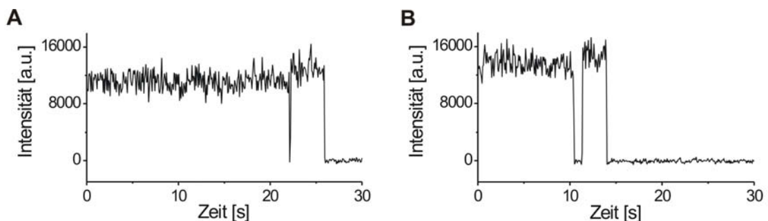
Abbildung 3.4.: Vereinzelt Blink-Ereignisse individueller Atto647-Farbstoffmoleküle. Durch den Übergang in einen Triplettzustand kann das Emissionssignal des Fluorophors für einen Zeitraum von wenigen Millisekunden (A) bis zu mehreren Sekunden (B) aussetzen.
