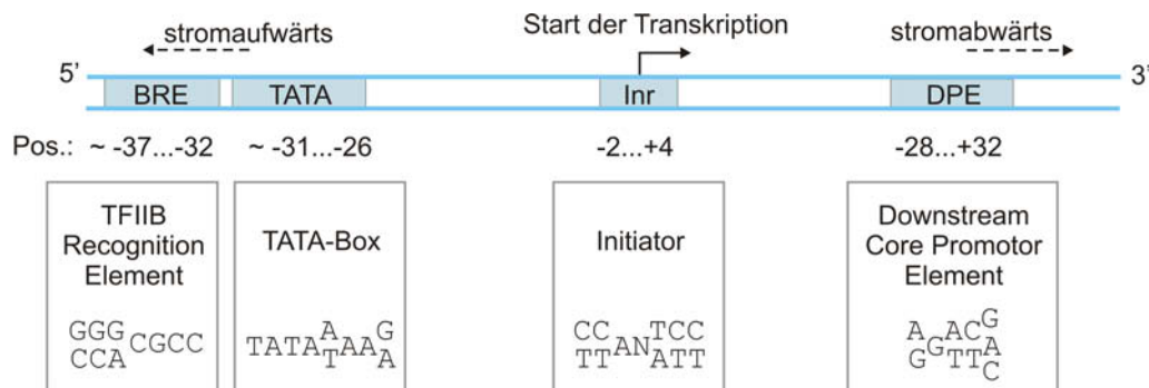
Abbildung 2.4.: Die Consensussequenzen von eukaryotischen Kernpromotoren. Gezeigt sind vier DNA-Sequenzmotive, die im Bereich des Transkriptionsstartpunktes liegen und zur Initiierung der Trankription beitragen. Diese Motive sind selten alle zusammen in einem Promotor vertreten. Vielmehr bestehen Promotoren meist nur aus zwei oder drei der vier Motive. In den erklärenden Boxen der einzelnen Motive sind die Consensussequenzen angegeben. Bei Positionen, für die alternative Sequenzen existieren, wurden die entsprechenden Basen übereinander angeordnet, wobei N für jede der vier Basen steht. Über den Box sind die Positionen der Sequenzen im Promotor angegeben. (Erstellt nach [20] und [9].)
