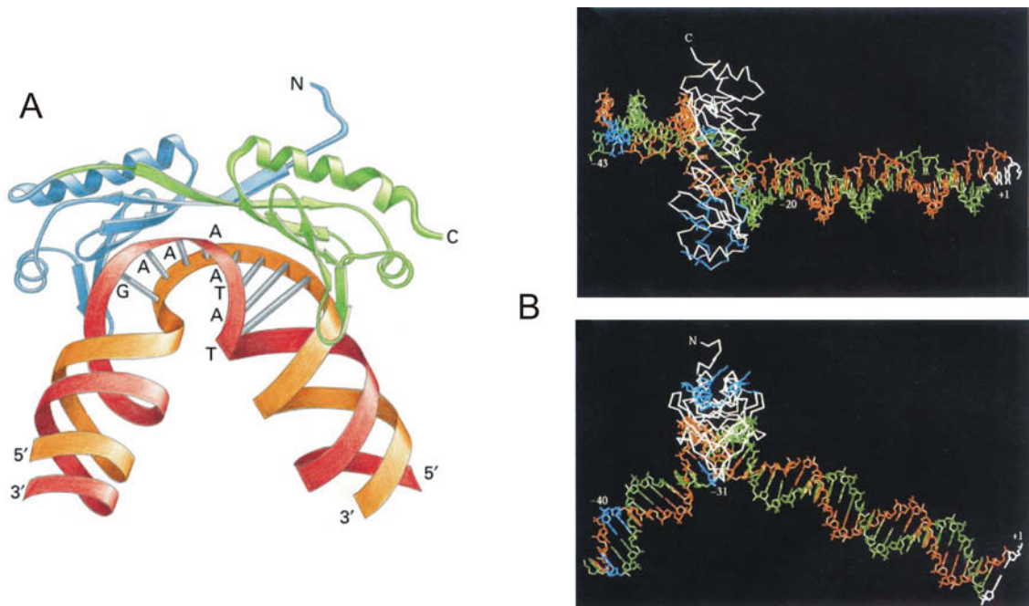
Abbildung 2.6.: Dreidimensionale Strukturen von DNA-gebundenem TBP: die C-terminale TBP-Domäne am Adenovirus Major Late Promoter (AdMLP). (A) Adaptierte Kristallstruktur, die zeigt, wie TBP in der kleinen Furche der TATA-Box bindet (der codierende DNA-Strang (rot) ist hier in 3'-5'-Richtung aufgetragen). Die zwei ähnlichen Strukturwiederholungen, welche die hoch konservierte DNA-Bindungsdomäne von TBP bilden, sind in blau (N-terminale Richtung) und grün (C-terminale Richtung) dargestellt (aus [9], Originalstruktur von Kim et al. [54]). (B) Kristallstrukturen vom TBP-AdMLP-Komplex, die die komplexen DNA-Konformationsänderungen aufgrund der TBP-Bindung zeigen [54] (TBP: weiße Bänder; codierender Strang: grün; Matrizenstrang: rot; Startpunkt der Transkription: weißes Basenpaar; Kontaktstellen zu TFIIA: blau). (oben) Knicke von jeweils knapp 90° stromauf- und -abwärts verursachen eine laterale Verschiebung des DNA-Doppelstranges von 18 Å. (unten) Der TBP-DNA-Komplex in einer um 90° gedrehten Ansicht. Die umfangreichen Verformungen der DNA an der TATA-Box führen zu einer Gesamtbeugung von ca. 80°, die zur Erkennung des aktivierten Promotors dienen könnte [32].
